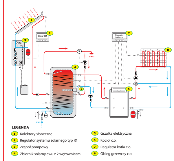
Solarna instalacja grzewcza do c.w.u. współpracująca z kotłem c.o. System solarny ze zbiornikiem cwu wyposażonym w 2 wężownice spiralne i grzałkę elektryczną
